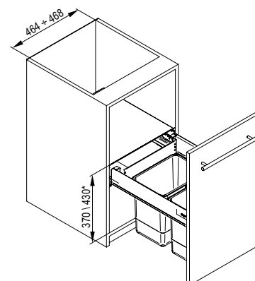
* подходит для высоты H=410
