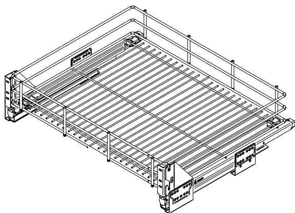
Товар в сборе
