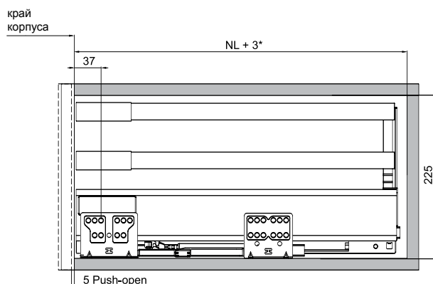
Ящик с креплением фасада
