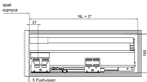
Ящик с креплением фасада
