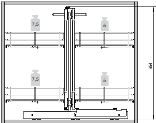
на рис. правый Corner Comfort
