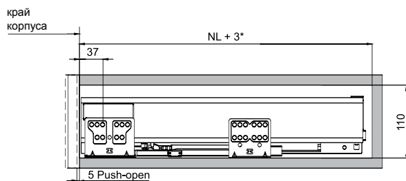
Ящик с креплением фасада
